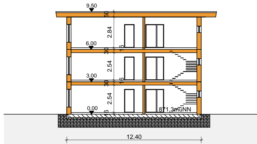
SCHNITT A-A
