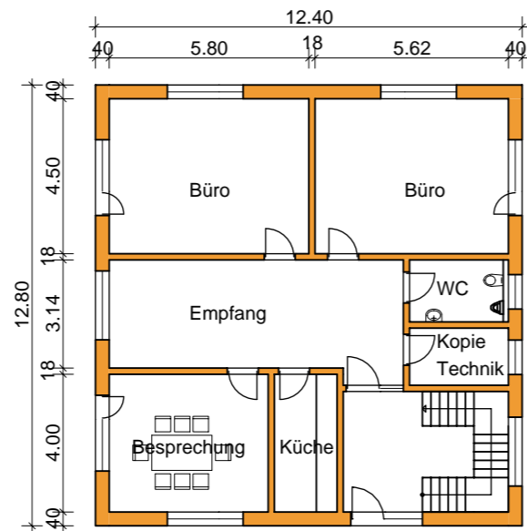
ERDGESCHOSS
